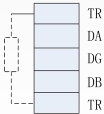
图 2 modbus 接口
