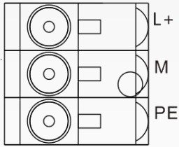
图 1 电源接口
